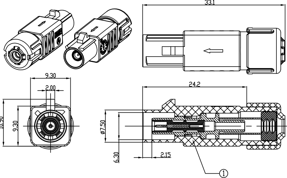
组装线缆后的连接器尺寸
